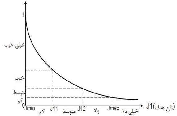
شکل (۳): نمونه‌ای از تابع درجه رضایت‌مندی برای یک مساله کمینه‌سازی.
