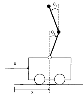
شکل (۸): سامانه‌ی گاری با پاندول معکوس دو لینکی.
