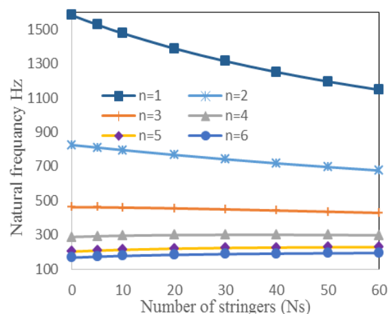
شکل (۷): تاثیر تعداد طولی بر روی فرکانس موده‌های محیطی
