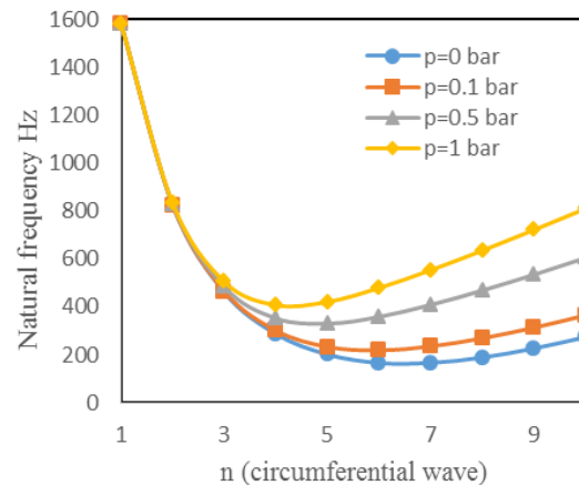
شکل (۱۰): بررسی تغییرات فشار داخلی استوانه بر روی فرکانس‌های طبیعی موده‌های محیطی استوانه.
