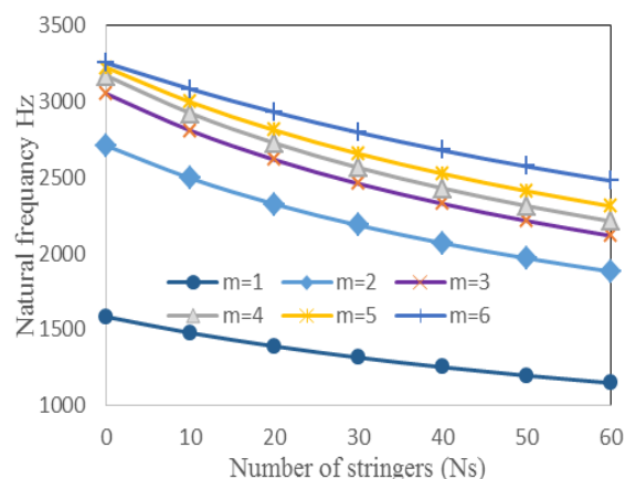
شکل (۶): تاثیر تعداد طولی بر روی فرکانس موده‌های محوری
