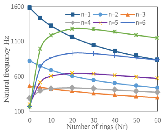
شکل (۹): تاثیر تعداد حلقوی‌ها بر روی فرکانس موده‌های محیطی
