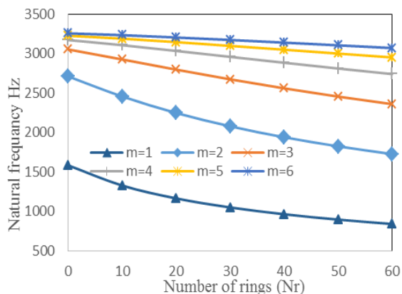
شکل (۸): تاثیر تعداد حلقوی‌ها بر روی فرکانس موده‌های محوری
