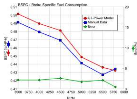
شکل (۱۱): مقایسه BSFC در مدل با داده‌های سازنده.
