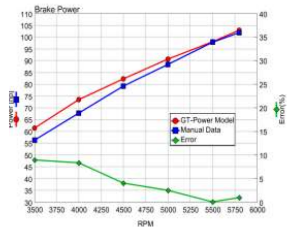
شکل (۷): مقایسه توان ترمزی در مدل با داده‌های سازنده.
