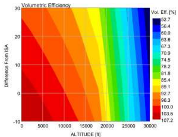
شکل (۳۵): کانتور راندمان حجمی بر حسب ارتفاع و دمای محیط
