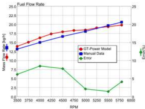
شکل (۹): مقایسه دبی سوخت در مدل با داده‌های سازنده.
