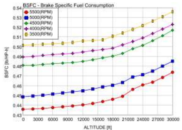
شکل (۲۰): تغییرات BSFC بر حسب ارتفاع در ۵ دور مختلف.
