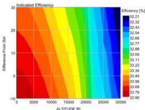
شکل (۳۴): کانتور راندمان اندیکاتور بر حسب ارتفاع و دمای محیط
