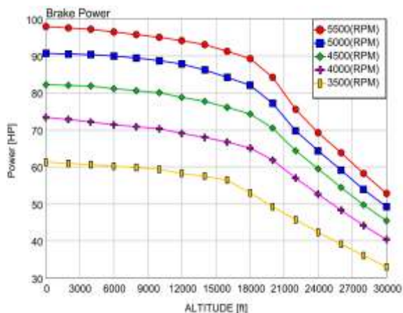
شکل (۱۹): تغییرات توان بر حسب ارتفاع در ۵ دور مختلف.
