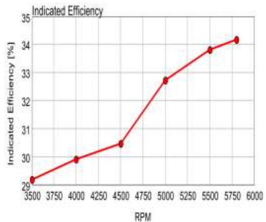
شکل (۱۷): راندمان اندیکاتوری بر حسب دور موتور در شرایط سطح دریا.
