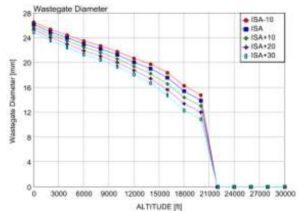
شکل (۲۹): میزان باز بودن دریچه کنار گذر بر حسب ارتفاع و دمای محیط.
