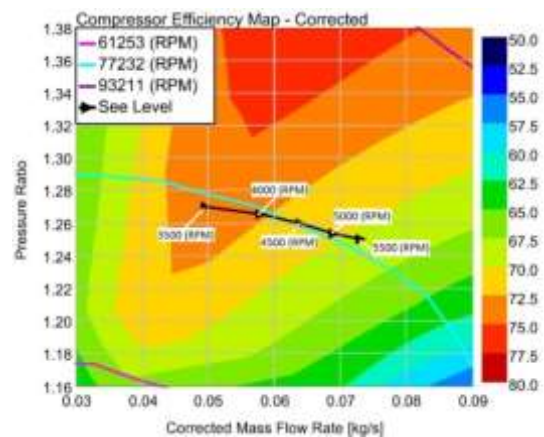
شکل (۱۸): نقاط کاری کمپرسور به تفکیک دور در ارتفاع سطح دریا.
