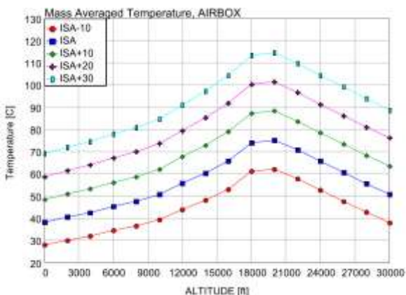
شکل (۳۳): تغییرات دمای هوای منیفولد ورودی بر حسب ارتفاع و دمای محیط.
