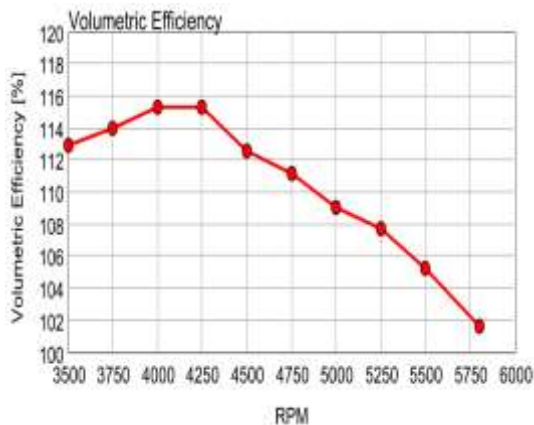
شکل (۱۶): راندمان حجمی بر حسب دور موتور در شرایط سطح دریا.
