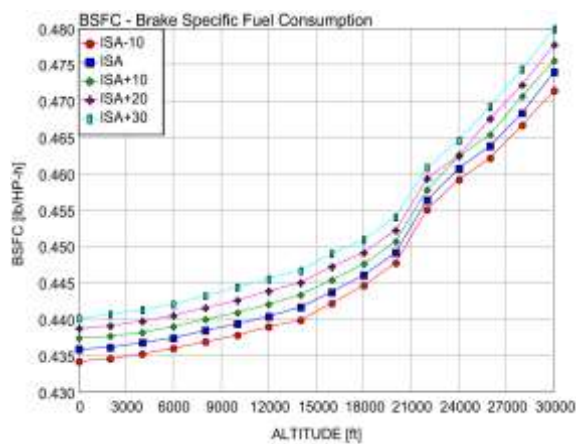
شکل (۳۱): تغییرات BSFC بر حسب ارتفاع و دمای محیط.
