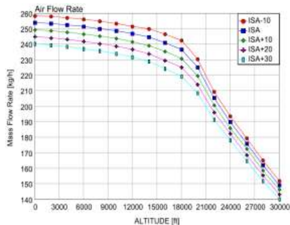
شکل (۲۸): تغییرات دبی هوای ورودی بر حسب ارتفاع و دمای محیط.
