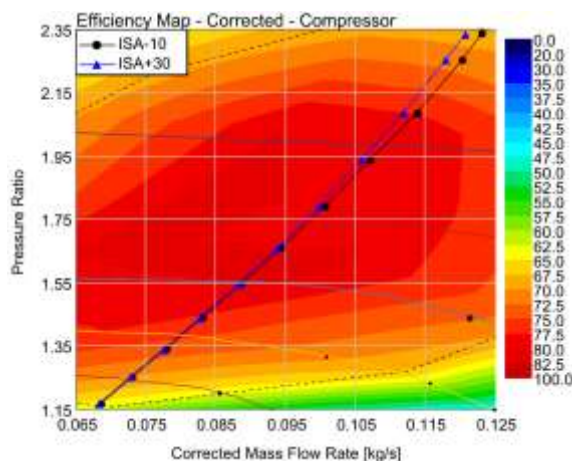
شکل (۳۲): خط کاری کمپرسور در دو دمای محیط مختلف در ۵۵۰۰ دور بر دقیقه.
