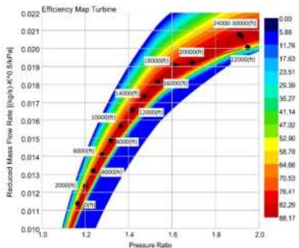
شکل (۲۶): خط کاری توربین در سرعت ۵۵۰۰ دور بر دقیقه در ارتفاعات مختلف.
