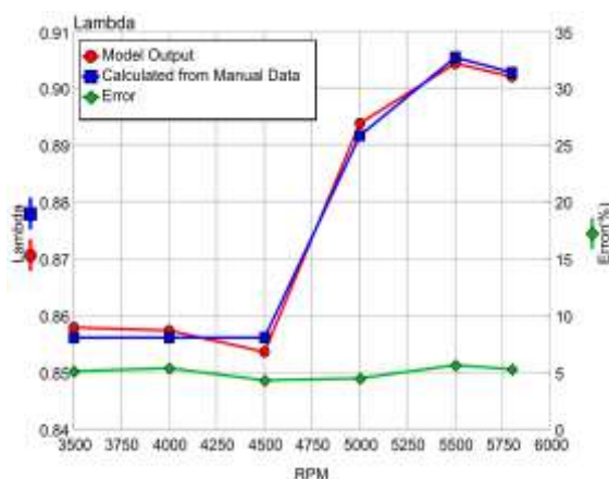
شکل (۱۰): مقایسه نسبت توازن مدل با مقدار محاسبه‌شده.
