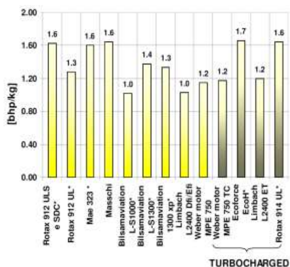
شکل (۲): مقایسه توان تولیدی به وزن موتور [۱].
