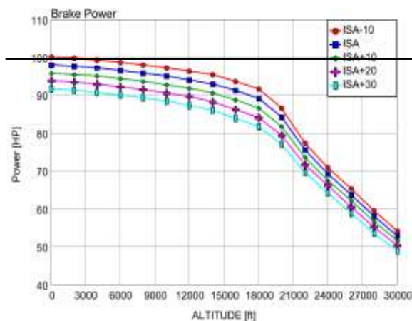
شکل (۲۷): تغییرات توان بر حسب ارتفاع و دمای محیط.
