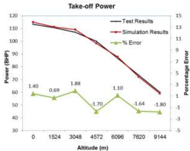
شکل (۴): توان تولیدی موتور روتکس ۹۱۴ بر حسب ارتفاع [۴].
