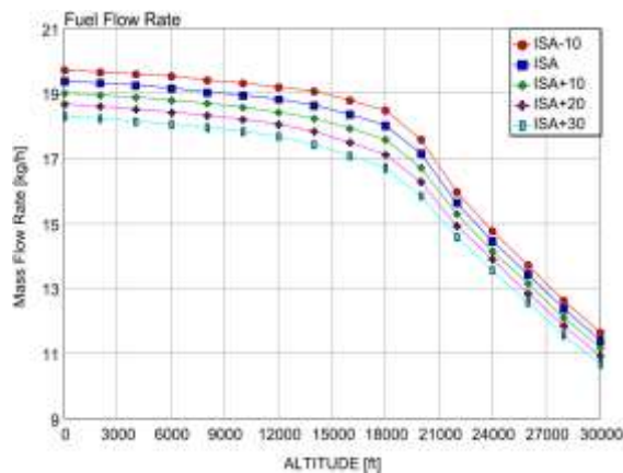
شکل (۳۰): تغییرات دبی سوخت بر حسب ارتفاع و دمای محیط.
