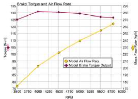
شکل (۱۵): گشتاور خروجی و دبی هوای موتور حاصل از مدل در شرایط سطح دریا.
