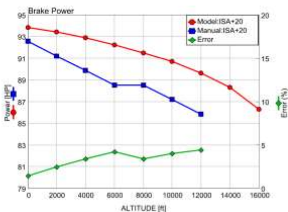
شکل (۱۴): مقایسه توان بر حسب ارتفاع در مدل و داده‌های سازنده در شرایط ISA+20.
