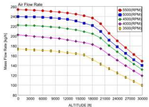
شکل (۲۱): تغییرات دبی هوای ورودی بر حسب ارتفاع در ۵ دور مختلف.
