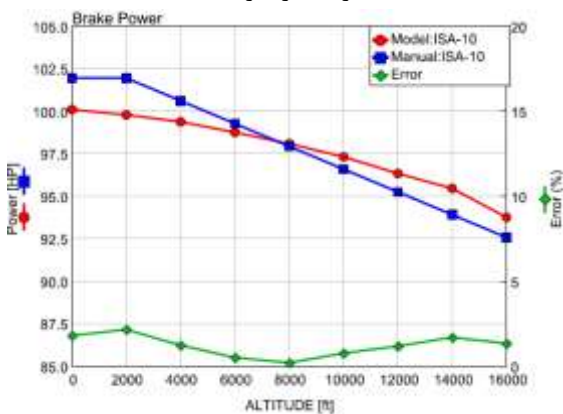
شکل (۱۳): مقایسه توان بر حسب ارتفاع در مدل و داده‌های سازنده در شرایط ISA-10.
