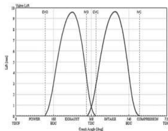
شکل (۵): پروفیل برخاست سوپاپ ورودی و خروجی.
