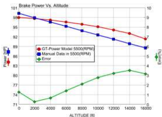
شکل (۱۲): مقایسه توان بر حسب ارتفاع در مدل و داده-های سازنده در شرایط ISA.
