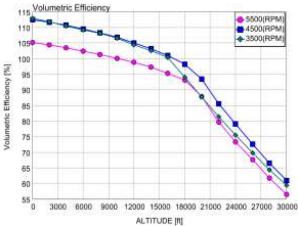
شکل (۲۲): تغییرات راندمان حجمی موتور بر حسب ارتفاع در ۳ دور مختلف.
