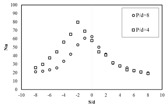
شکل (۸): تاثیر تعداد جت بر توزیع عدد ناسلت
