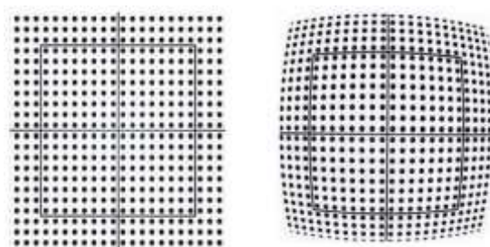
شکل (۱۱): استفاده از یک الگو نقطه ای برای کالیبراسیون دوربین.
