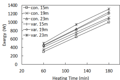
شکل (۱۰): تغییرات زمانی اگزرژی نسبت به طول لوله چگالنده در هر دو حالت دارای چگالنده با قطر ثابت و متغیر.
