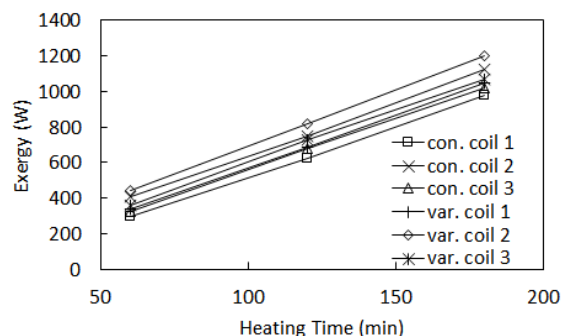
شکل (۱۲): تغییرات زمانی اگزرژی با تغییر قطر در هر دو حالت دارای چگالنده با قطر ثابت و متغیر.
