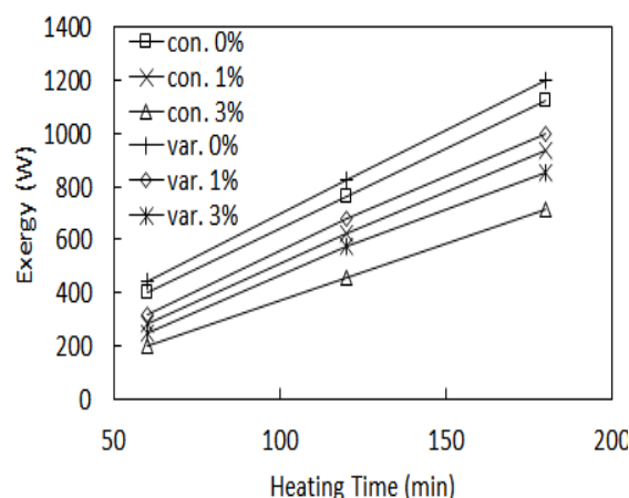
شکل (۸): تغییرات زمانی اگزرژی در هر دو چگالنده قطر ثابت و متغیر در غلظت‌های مختلف نانولوله کربنی درون دیواره لوله مسی چگالنده.
