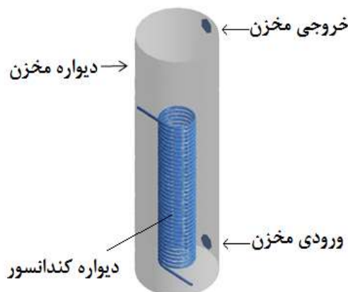
شکل (۱): شرایط مرزی اعمال شده بر مخزن آب.
