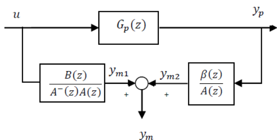
شکل (۲): بلوک دیاگرام پیش‌بینگر مدل تجزیه شده به سامانه‌های پایدار.
