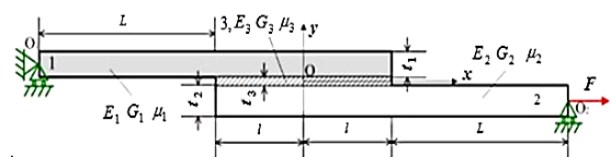
شکل (۱): مدل دو بعدی اتصال تک‌لبه.
