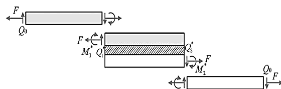
شکل (۲): نمودار تعادل نیرویی اتصال تک لایه [۱۵].
