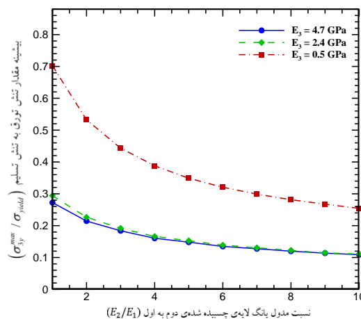
شکل (۸): مقایسه استحکام سه نوع چسب در اتصال نامتقارن.
