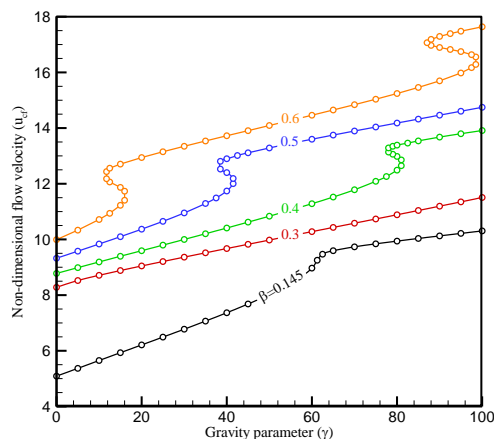
شکل (۹): تغییرات سرعت بحرانی بی‌بعد بر حسب پارامتر بی‌بعد گرانش \gamma و مقادیر مختلف پارامتر جرم \beta .
