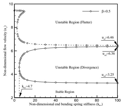
شکل (۷): تغییرات سرعت بحرانی بی‌بعد بر حسب سختی بی‌بعد فنر خمشی انتهایی برای یک لوله یکسرگیردار با \beta = 0.5 .
