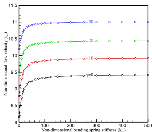
شکل (۸): تغییرات سرعت بحرانی بی‌بعد بر حسب سختی بی‌بعد فنر خمشی ابتدایی، k_{sp} ، برای یک لوله یکسره مفصل با مقادیر مختلف \gamma و \beta = 0.5 .
