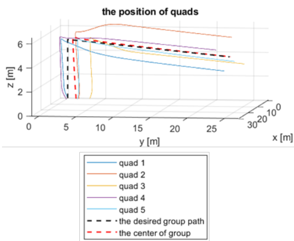
شکل (۴): موقعیت سه‌بعدی حرکت گروهی چهارپره‌ها
