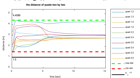
شکل (۵): نمودار فاصله دوه‌دو چهارپره‌ها
