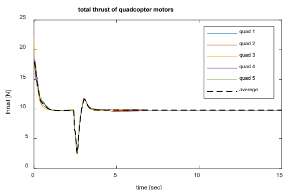
شکل (۸): نیروی بالابرنده هر چهارپره
