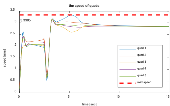
شکل (۶): سرعت چهارپره‌ها
