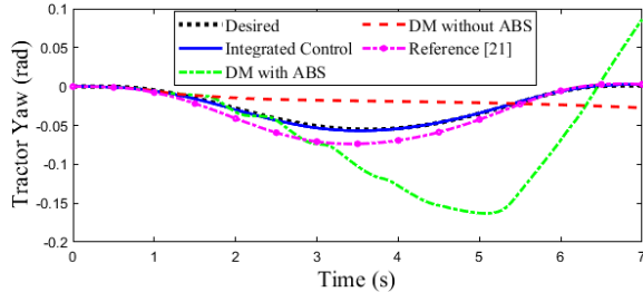
شکل (۷): زاویه چرخش کشنده.
