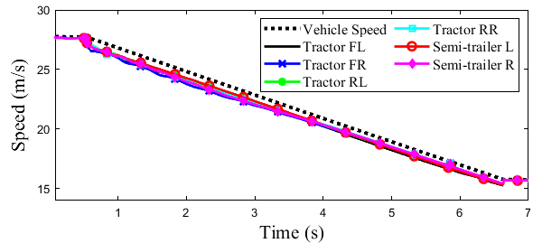
شکل (۱۶): سرعت چرخ‌های خودروی کنترل‌شده.
