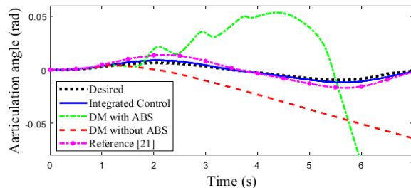
شکل (۸): زاویه مفصل.
