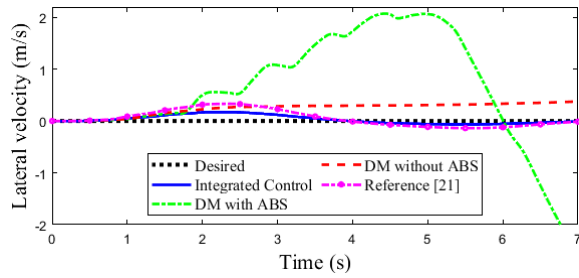
شکل (۹): سرعت جانبی کشنده
