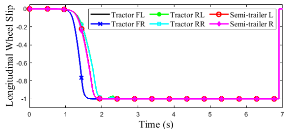
شکل (۱۱): لغزش طولی تایرهای خودروی حالت اول.
