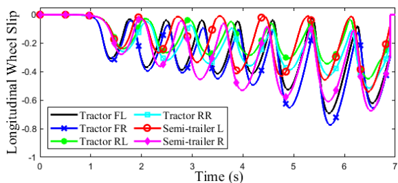
شکل (۱۳): لغزش طولی تایرهای خودروی حالت دوم.
