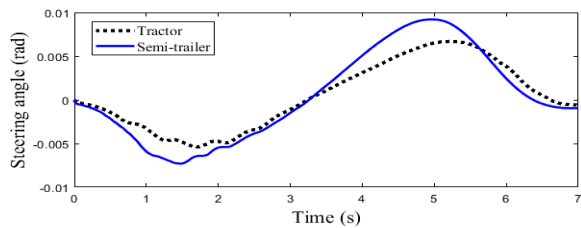
شکل (۱۸): زاویه فرمان چرخ‌های کشنده و نیم‌تریلر.
