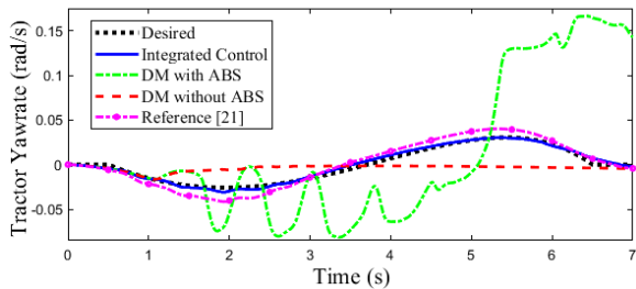
شکل (۱۰): نرخ زاویه چرخش کشنده
