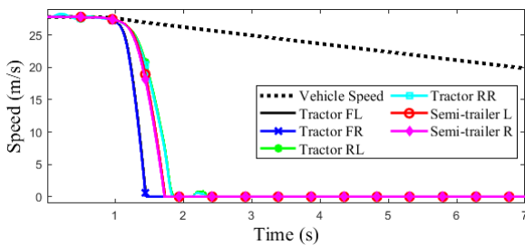
شکل (۱۲): سرعت چرخهای خودروی حالت اول.
