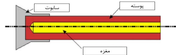
شکل (۱): شماتیک پرتابه پله [۱].
