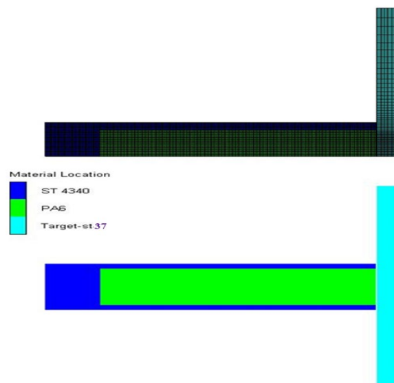
شکل (۹): هندسه پرتابه و هدف.
