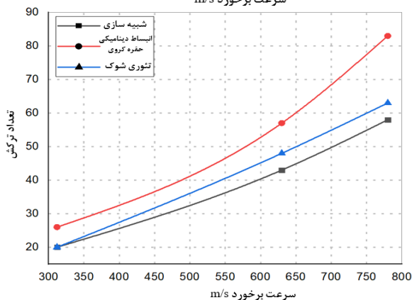
شکل (۱۲): ضخامت حد بالستیک و تعداد ترکش (ضخامت
