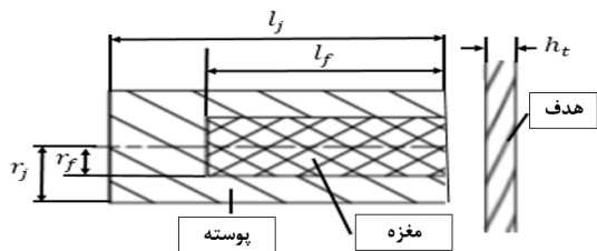
شکل (۳): شماتیک پرتابه و هدف.
