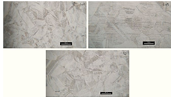
شکل (۴): ریزساختار نمونه‌های فولاد آلیاژی زنگ‌نزن L ۳۰۴ برحسب پاس‌های انجام‌شده در فرایند پرس کاری شیارمقید: الف) نمونه اولیه آنیل شده؛ ب) نمونه تک پاسه؛ ج) نمونه سه پاسه.
