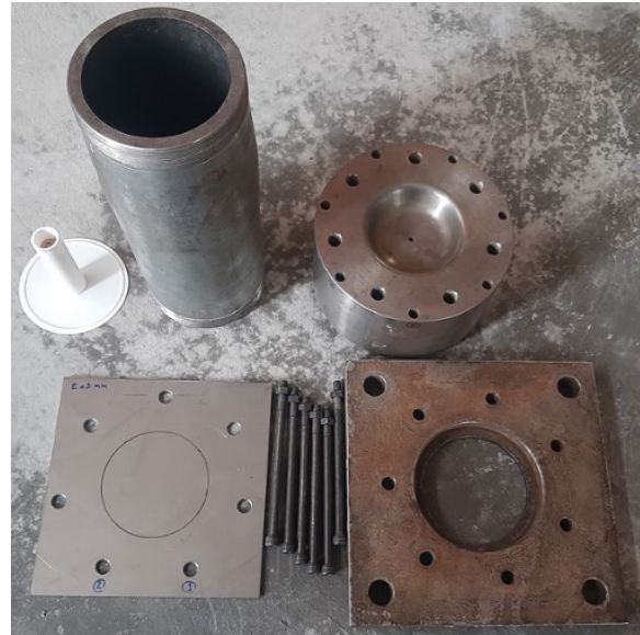
شکل (۴): نمایی از تجهیزات آزمایشگاهی شامل قالب مادگی، ننگه‌دارنده، لوله انفجار، نمونه ورق.
