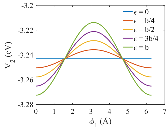
شکل (۶): انرژی پتانسیل گریز از مرکز برحسب زاویه انحراف و به ازای موقعیت‌های مختلف مولکول باکی‌بال.
