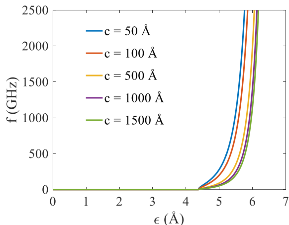
شکل (۱۲): تأثیر شعاع حلقه نانوتورس بر فرکانس نانوونسانگر باکی‌بال-نانوتورس.
