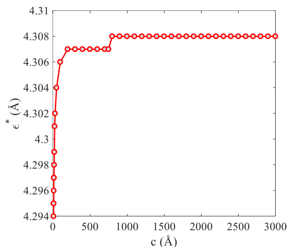
شکل (۵): موقعیت تعادل مولکول باکی‌بال برحسب شعاع حلقه نانوتورس.
