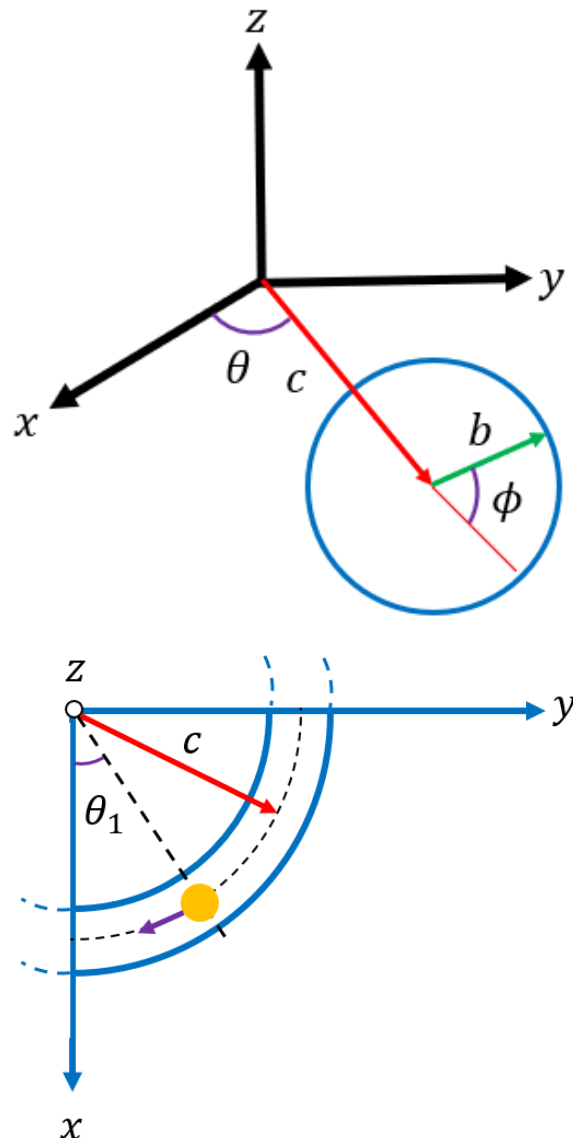
شکل (۲): هندسه نانوتورس.
