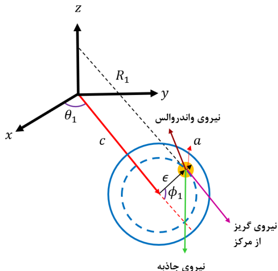
شکل (۱): هندسه نانونوسانگر باکی‌بال-نانوتورس به همراه نیروهای اعمال شده به باکی‌بال.
