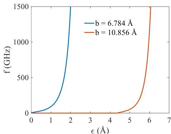
شکل (۱۱): تأثیر شعاع لوله نانوتورس بر فرکانس نانوسانگر باکی‌بال-نانوتورس.
